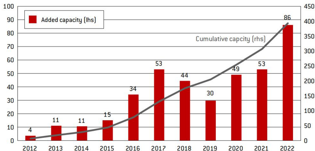
图 20 太阳能光伏装机容量增长，中国，GW
