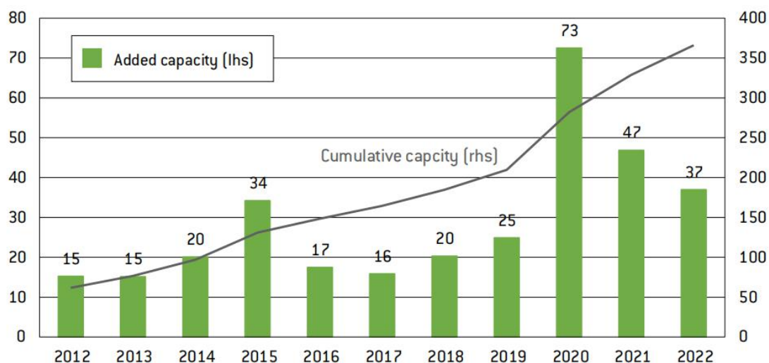
图 21 风电装机容量增长，中国，GW
