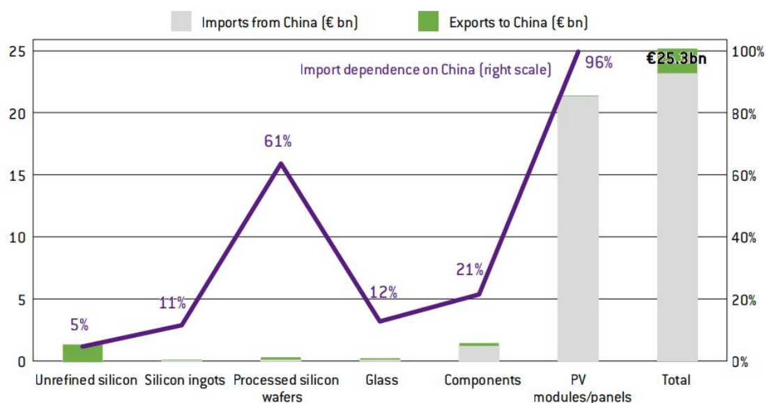
图 6 2022 年欧盟在太阳能光伏供应链中对中国的依赖
