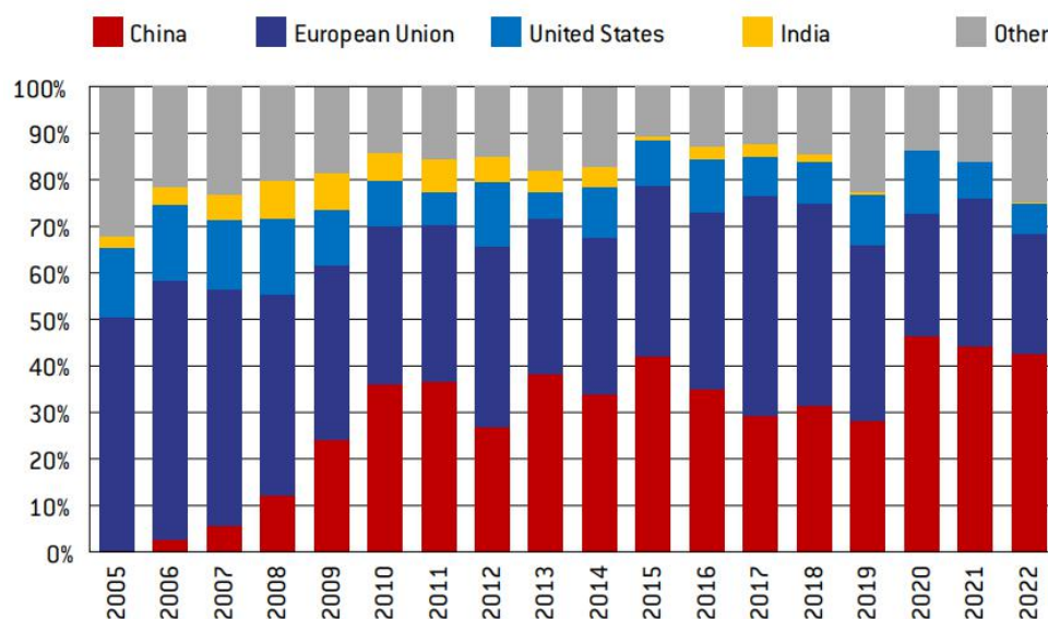
图 11 全球风机制造份额
