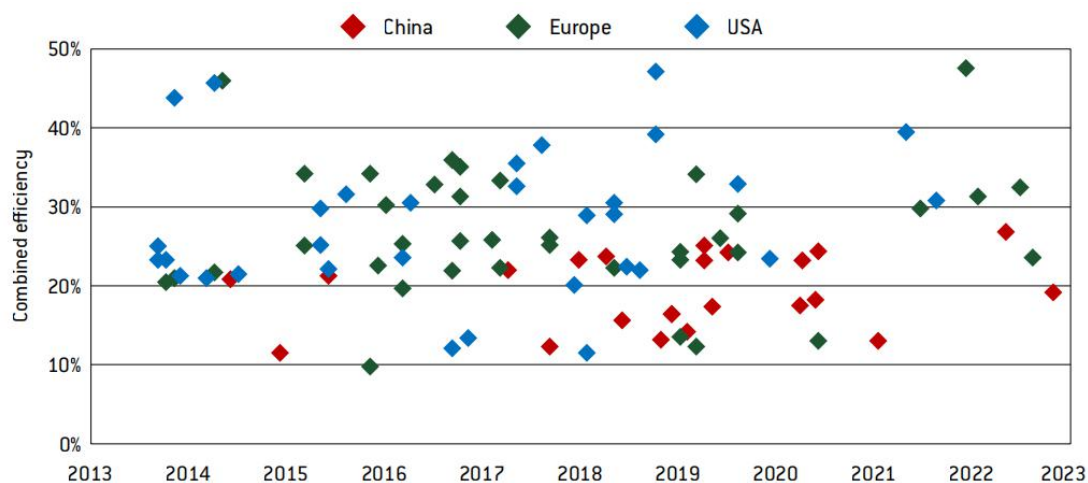
图 7 所有技术的太阳能光伏效率记录（欧盟、美国、中国）
