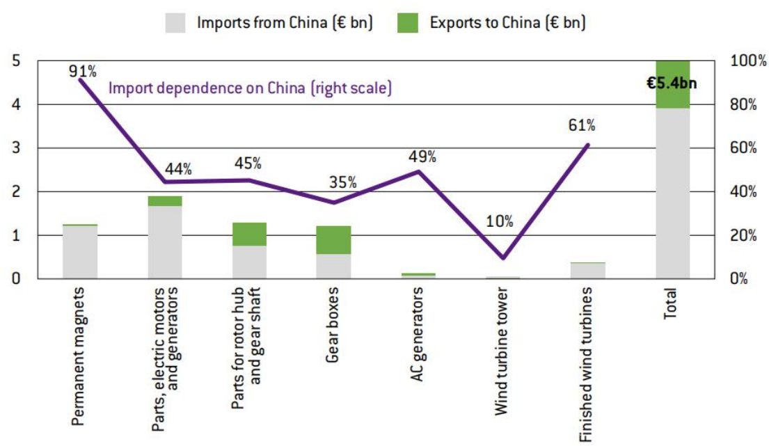
图 12 欧盟在风机供应链中对中国的依赖（2022 年）
