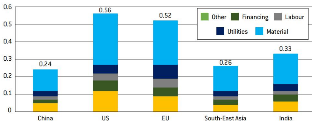
图 22 每个地区的太阳能光伏组件制造成本，美元/瓦
