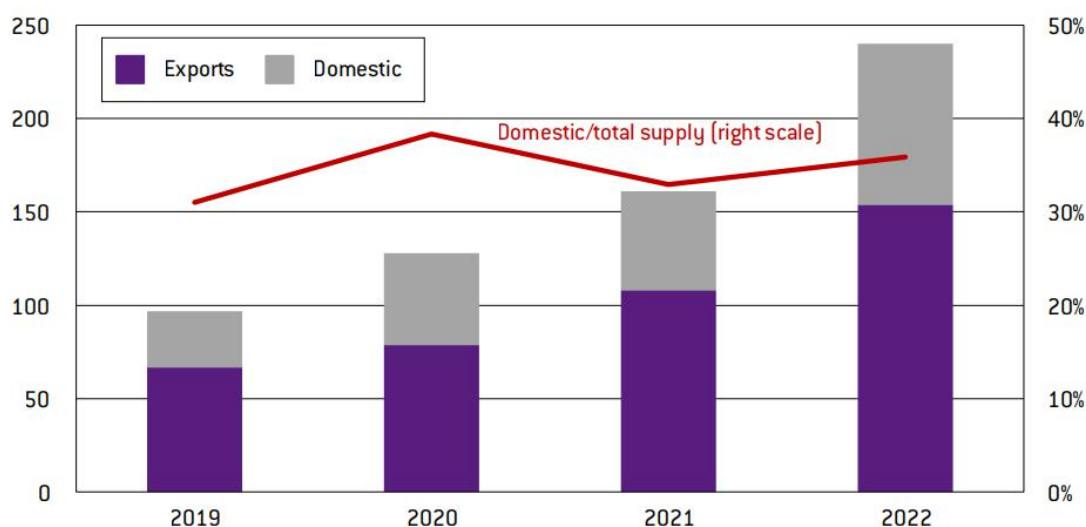
图 19 中国太阳能光伏出口与国内安装，GW
